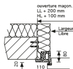
Cadre Thermotec maçonnerie
