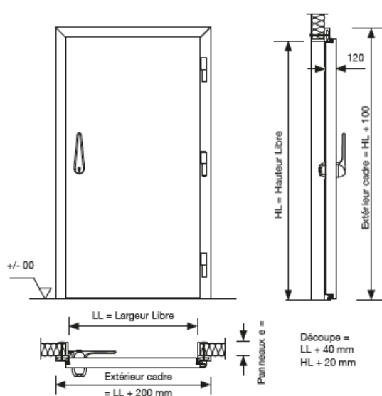
Cadre PVC 100x40 habillage px
