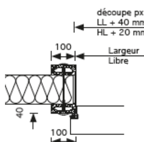
Cadre PVC 100x40 contre-cadre PVC
