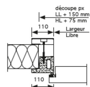
Contre-cadre Thermotec montage px
